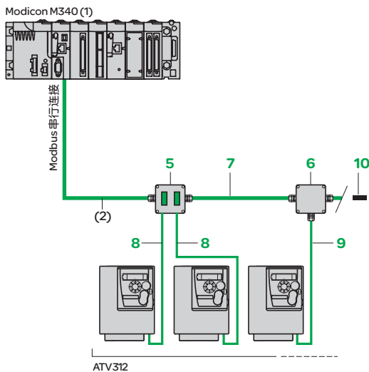
通过分管连接的Modbus串行连接架构示例
