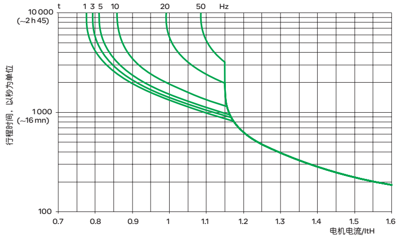
电机热保护曲线
