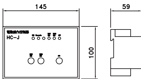
外型圖
